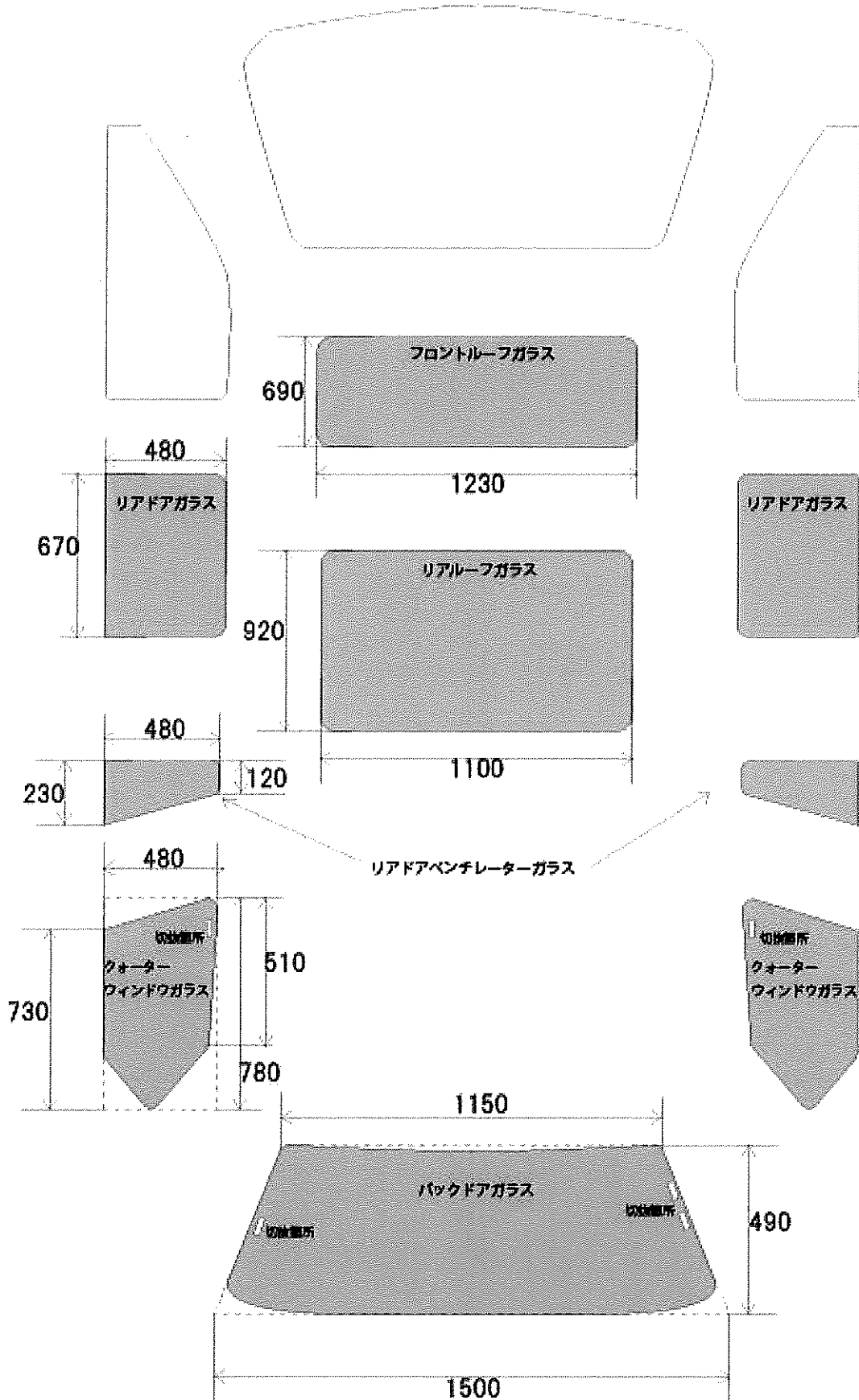
図1 フィルムの施工箇所及びガラスの寸法 (mm)
